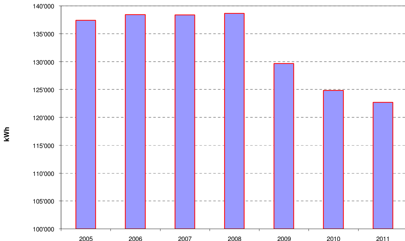
Illuminazione pubblica - evoluzione del consumo in kWh dal 2005 al 2011
